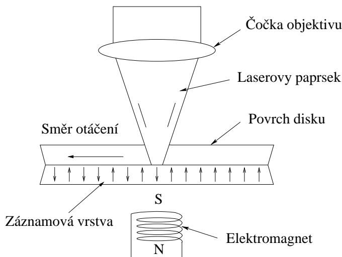
Obrázek 8: Záznam dat u magnetooptických disků
