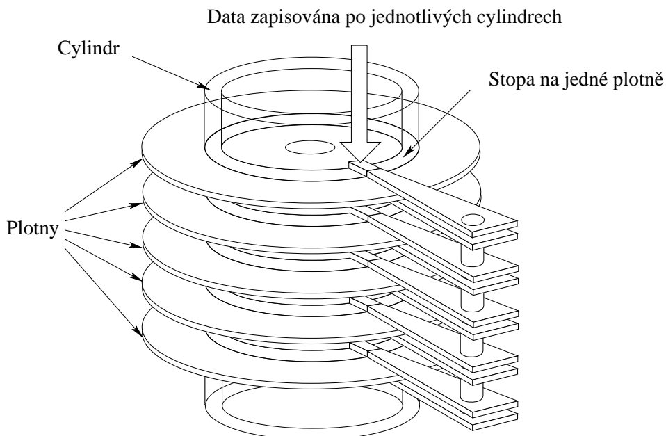
Obrázek 2: Cylindry
