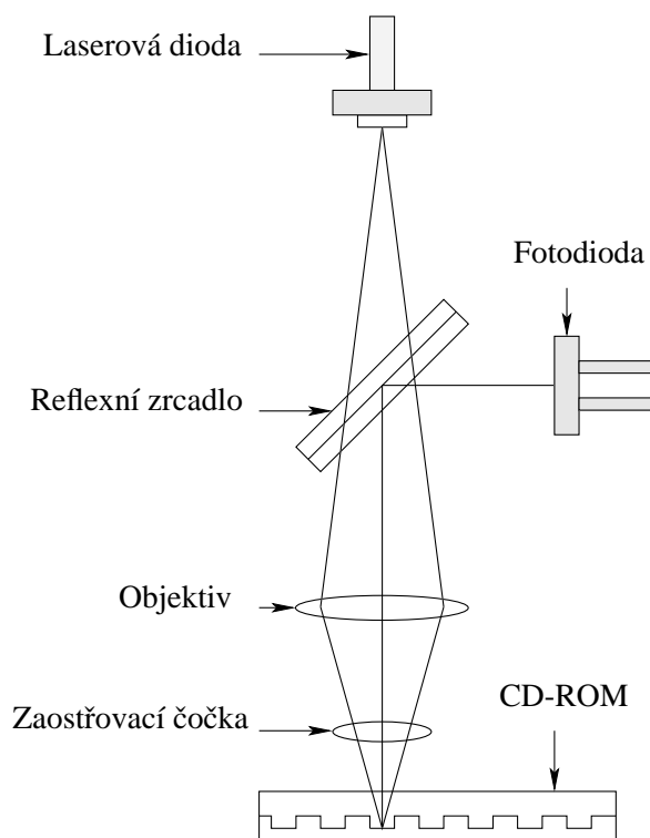
Obrázek 5: Princip optického záznamu
