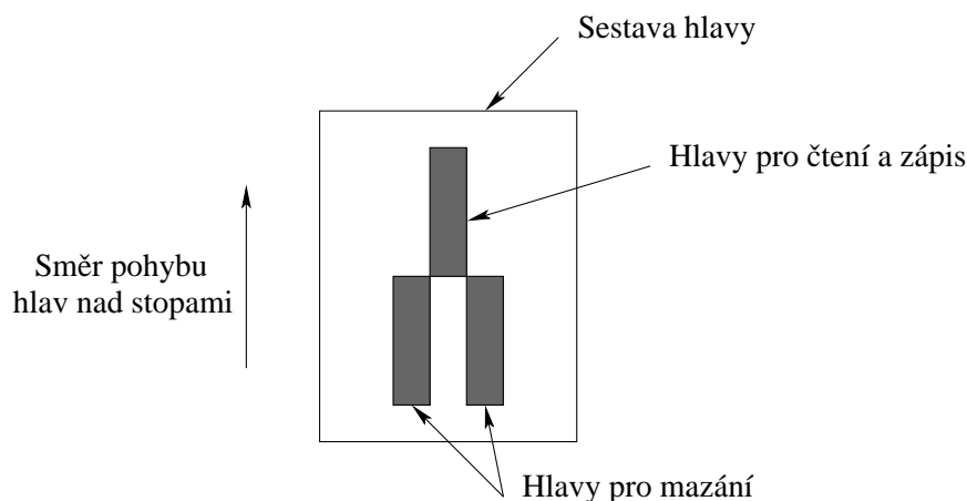
Obrázek 4: Sestava hlavy disketové mechaniky
