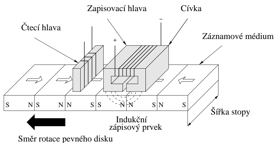
Obrázek 1: Princip magnetického zápisu
