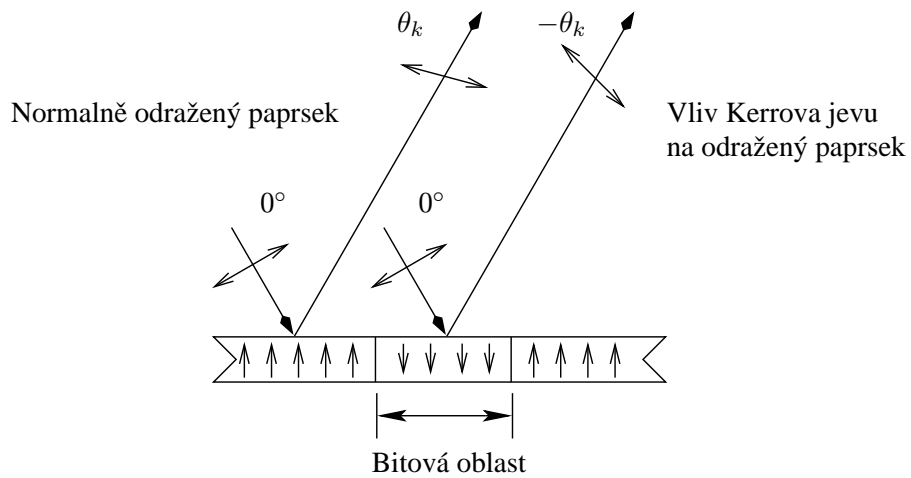
Obrázek 9: Kerrův efekt
