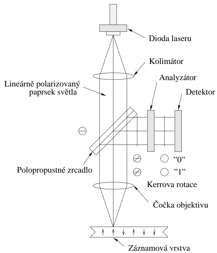
Obrázek 10: Čtení dat u magnetooptických disků
